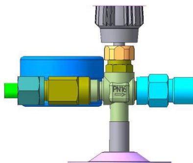
Рис 2.К-1101-16М DN1,6 ДЖЕТ 000 270 000-20
