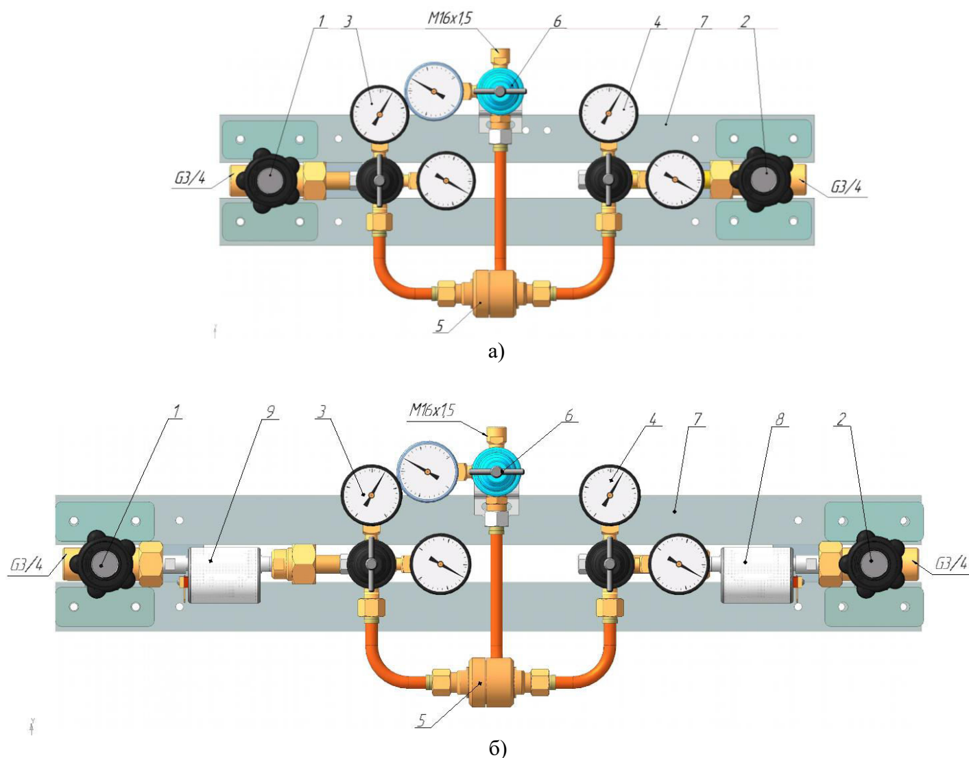
Рис.1 Щит автопереключения плеч перепускных газовых рам.
