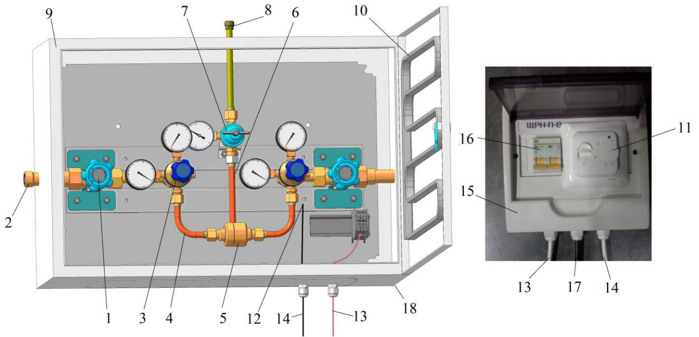
Рис.1а Щит автопереключения газовых рампов закрытого типа в термобоксе исп. ДЖЕТ 653 00 00 00.
