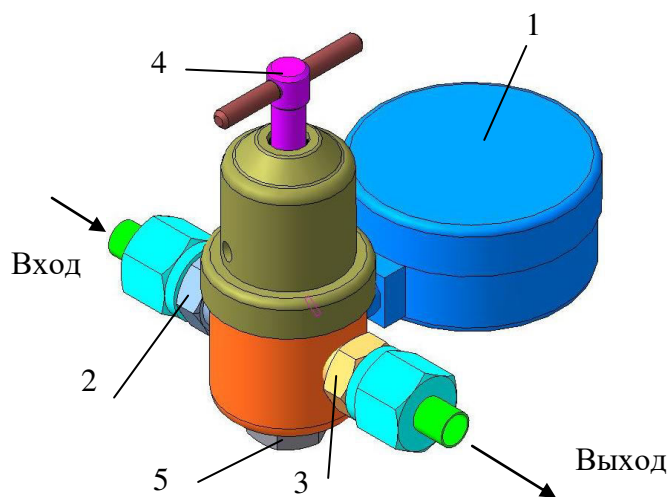
Рис1 Редуктор СУО-10
