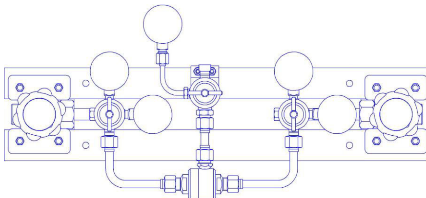
Рис.2. Щит автопереключения
