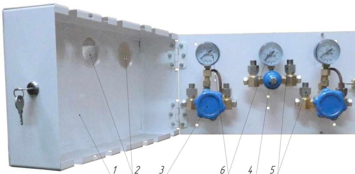
Рис.1 Коробка поэтажная отключающая УГВ4/3 (два клапана и сетевой редуктор) 1- корпус; 2 - смотровые окошки; 3 - клапан запорный К1412-16; 4 - редуктор сетевой СКО-10 или СУО-10; 5 - штуцера входа и выхода газа; 6 - манометр.
