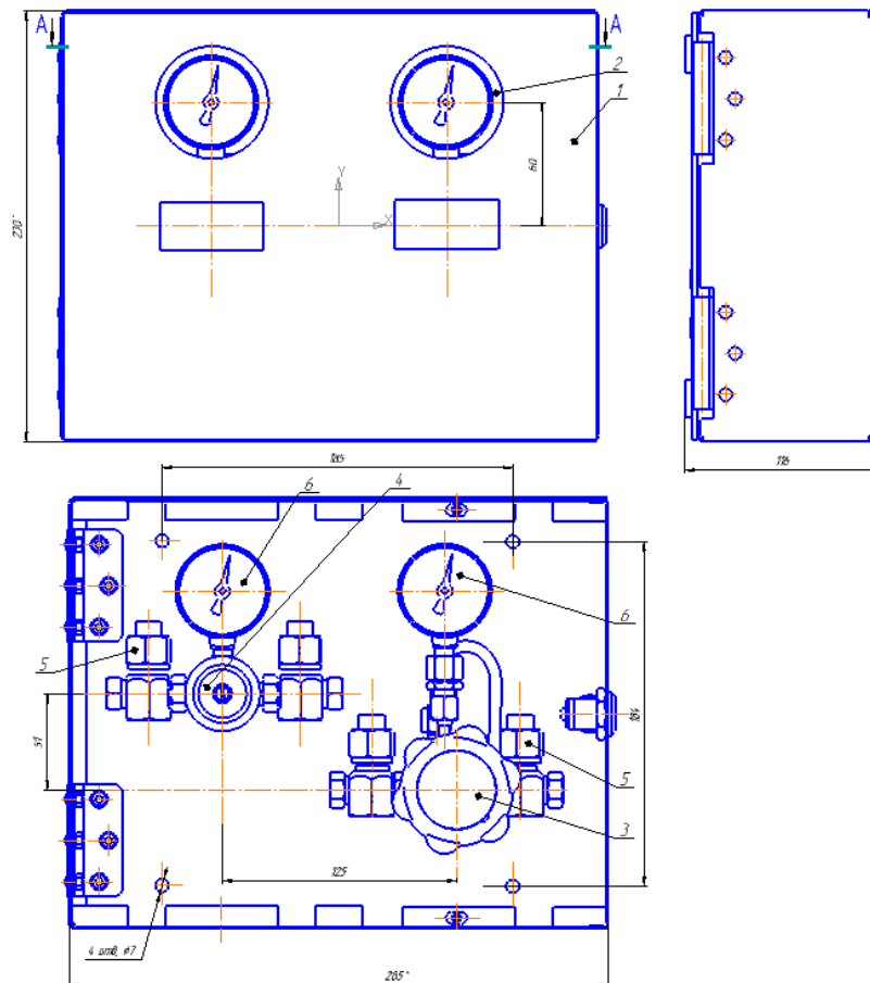
Рис.1 Коробка поэтажная отключающая УГВ4/2 (сетевой редуктор и клапан)
