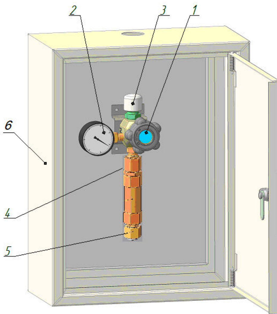
Рис.1 Пост газоразборный ПГК-35-з
