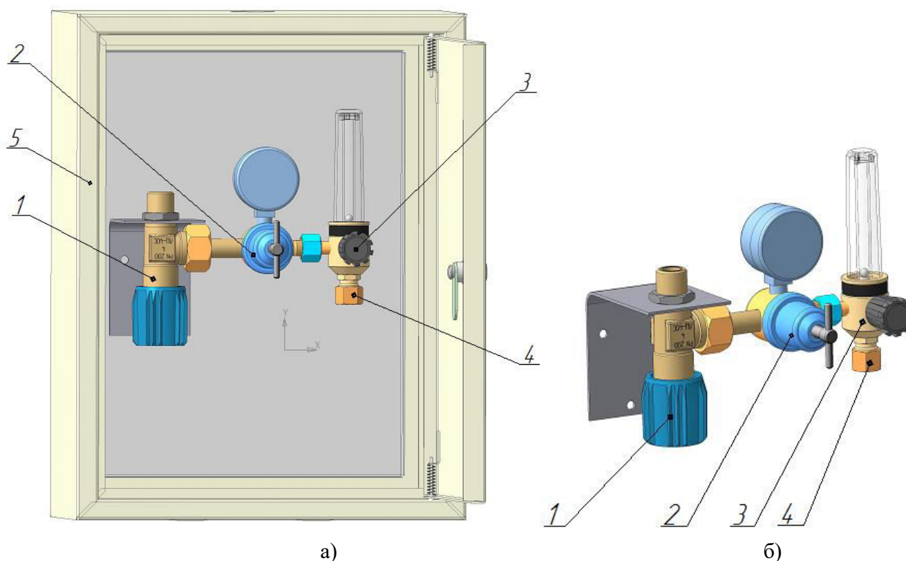
Рис. 1. Посты газоразборные: а - ПГАр-25РТ-з; б - ПГАр-25РТ 1 - клапан; 2 - редуктор; 3 - ротаметр с регулятором; 4 - заглушка; 5 - бокс
