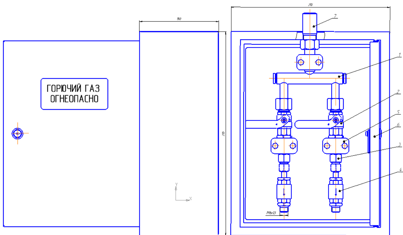
Рис. 1. Пост газоразборный ПГГ-10з-2
