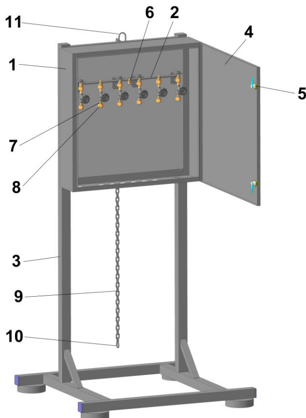
Рис. 1. Пост газопитания
