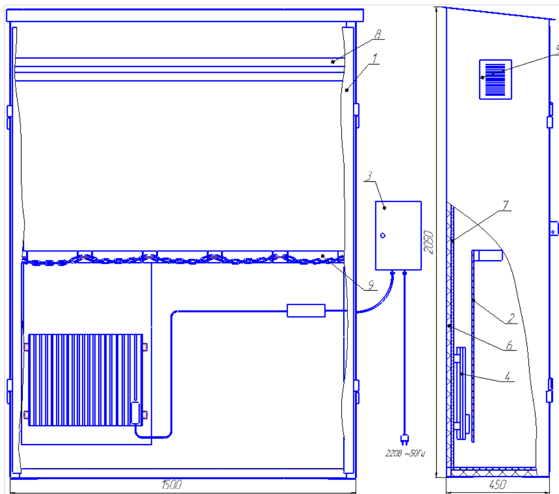
Рис.1 Общий вид термошкафа для газовых баллонов.
