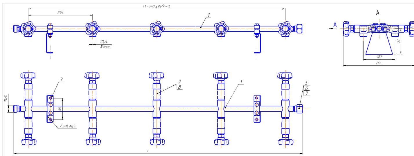
Рис.1 Коллектор рамповый КР-02 ДЖЕТ 556 24 01 00
