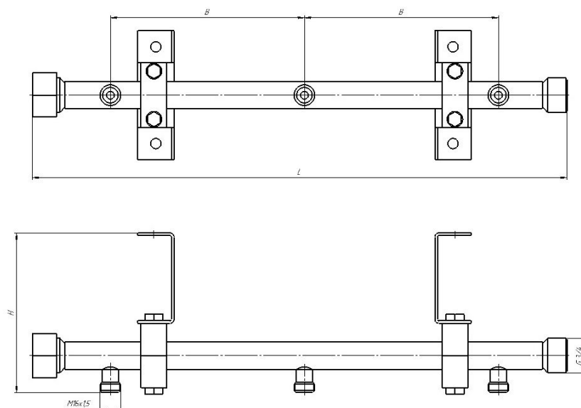
Рис.1 Коллектор газовый КР-03 ДЖЕТ 34 00 00 00
