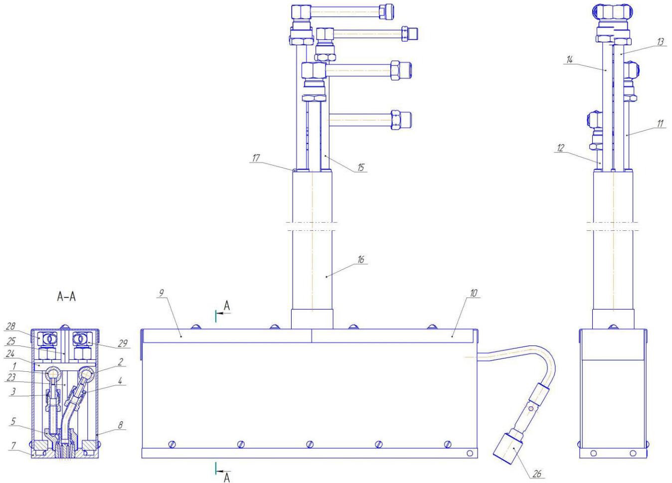
Рис.2 Чертеж горелки
