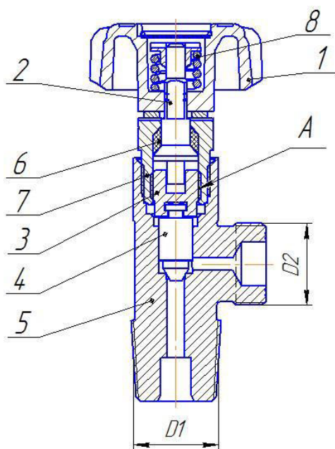
Рис. 3 Устройство вентиля
