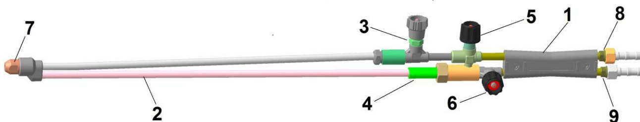
Рис. 2 Резак РЗПГсб (L=1300, 1500 мм)
