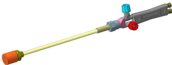
Рис.2 Горелка ГП-1 Шторм
