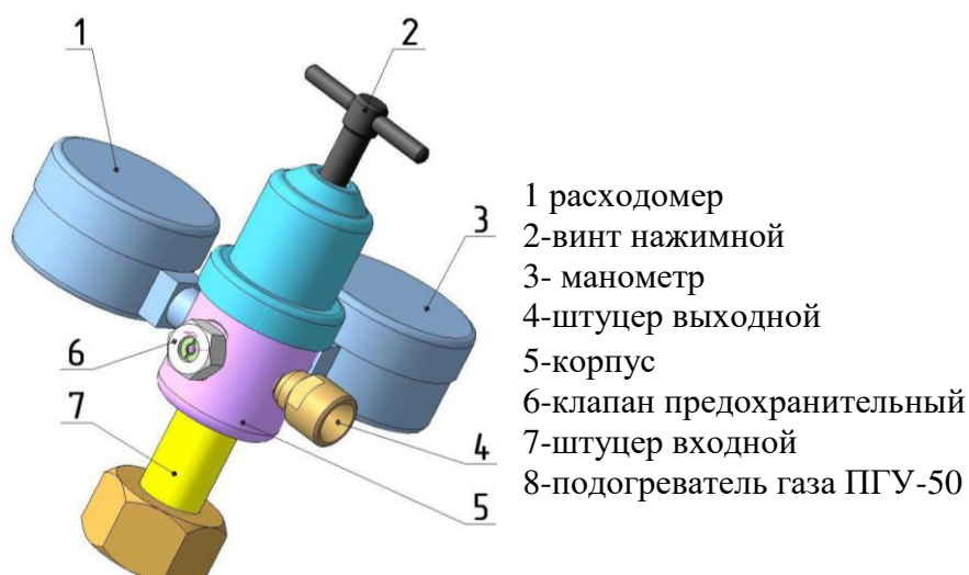
Рис.1 Регулятор расхода газа У-30
