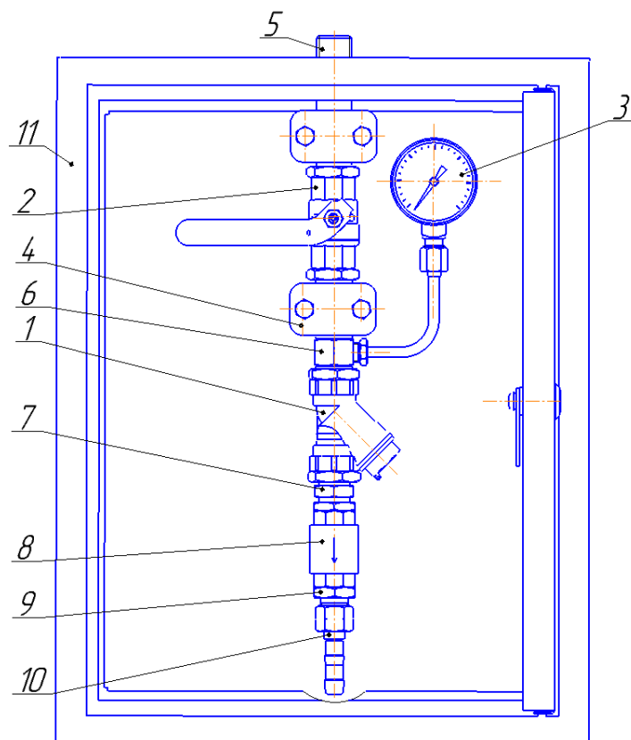
Рис. 1. Пост газоразборный ПГГ-10-з
