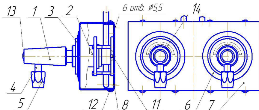
Рис.1 СКБ-1 ДЖЕТ 378 00 00 00
