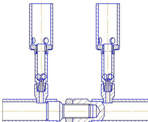
Рис.2 Соединение горелок
