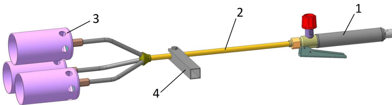
Рис.1 Горелка модели ГВ ДЖЕТ 119 16 1- ствол; 2- удлинитель; 3- наконечник; 4-рукоятка
