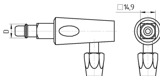
Рис.3 Штекер газовой ДЖЕТ 294 01 00 00-03;-04
