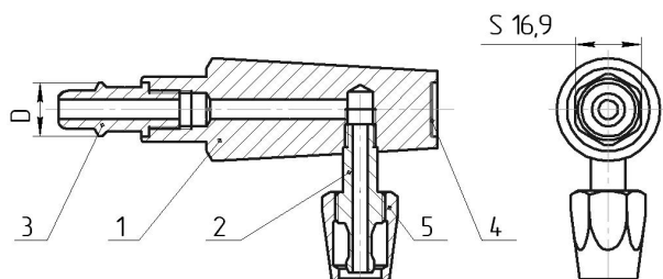
Рис.1 Штекер газовой ДЖЕТ 294 01 00 00;-01
