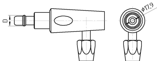
Рис.2 Штекер газовой ДЖЕТ 294 01 00 00-02
