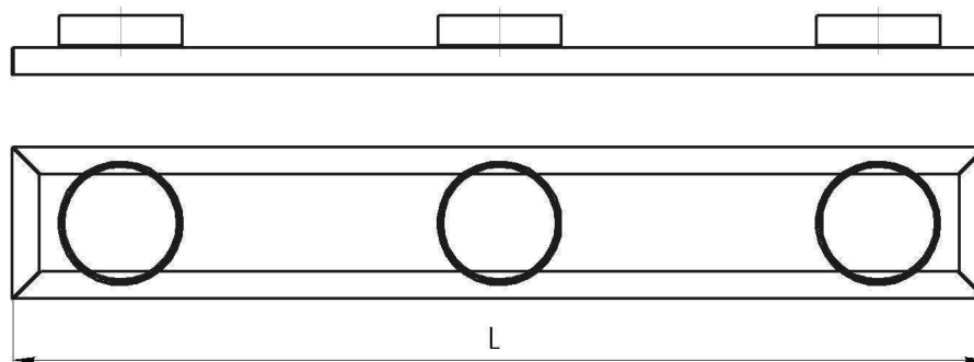
Рис.1 Подставка ДЖЕТ 214 03 00 00
