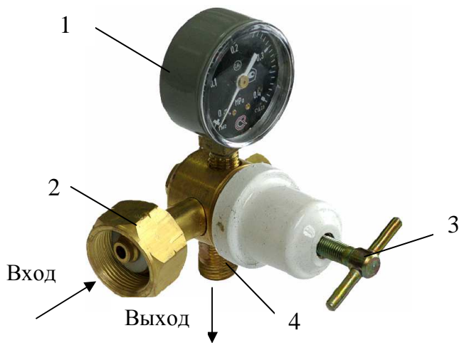
Рис. 1 Редуктор САО-10 ДЖЕТ 279 00 00 00
