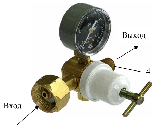
Рис.2 Редуктор САО-10 ДЖЕТ 279 00 00 00-01
