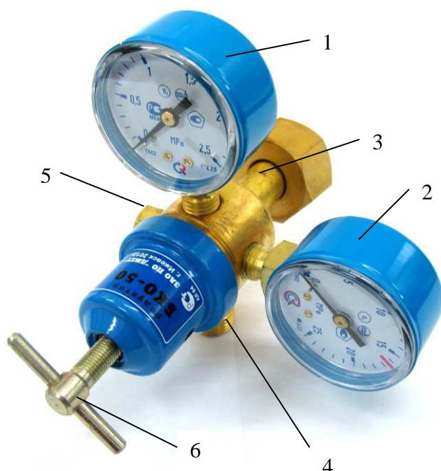
Рис.1 Редуктор БКО-50
