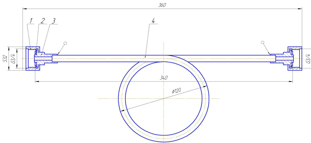
Рис. 2 Змеевик ЗМК ДЖЕТ 133 00 00 00-03 1- гайка накидная; 2 – прокладка; 3 – переходник; 4 - трубка
