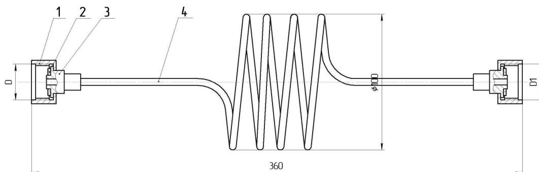
Рис.1 Змеевик ЗМК.
