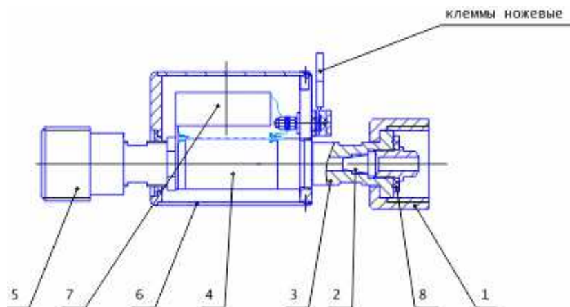
Рис.1 Подогреватель газа ПГУ-50
