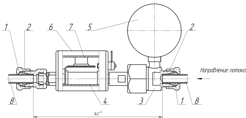
Рис. 1. Подогреватель универсальный ПГУМ-50.
