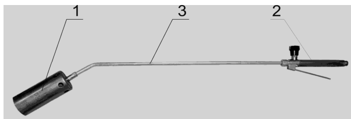
Рис.1 Горелка модели ГВ ДЖЕТ 119-30, ГВ ДЖЕТ 119-31, ГВ ДЖЕТ 119-33, ГВ ДЖЕТ 119-35
